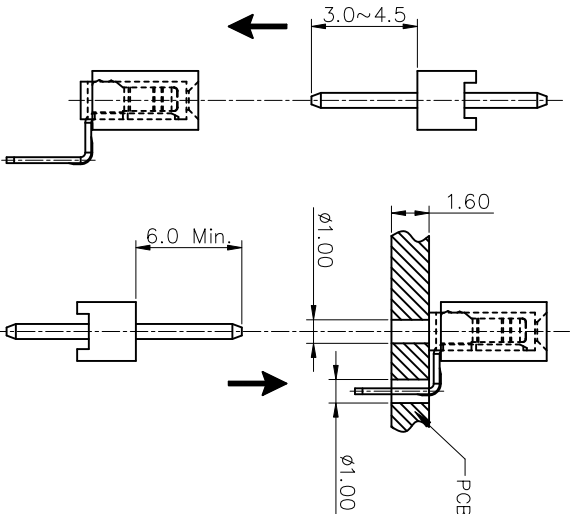
TOP INSERT
