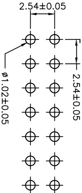
P.C.B. LAYOUT
