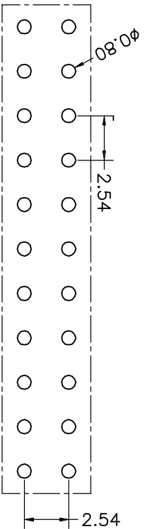
P.C.B LAYOUT
