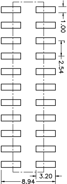
P.C.B LAYOUT
