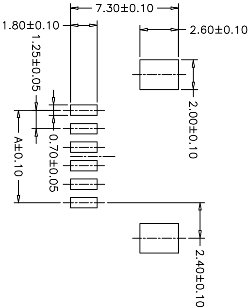
P.C.B. LAYOUT
