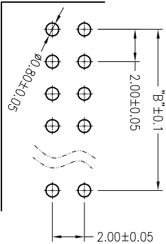
P.C.B LAYOUT
