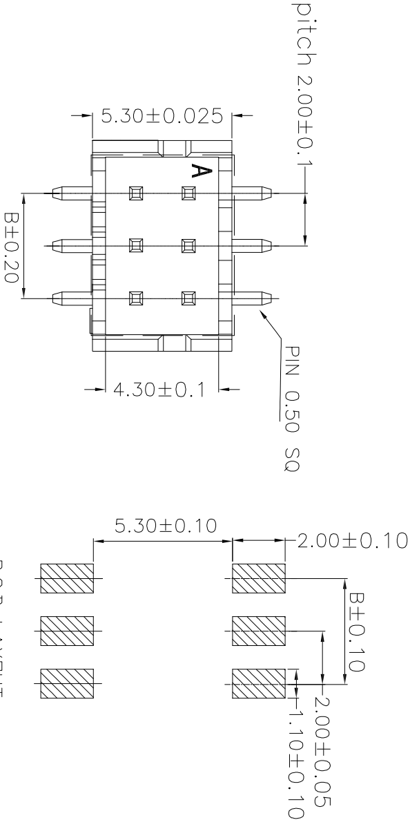
P.C.B LAYOUT
