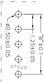
P.C.B. LAYOUT
