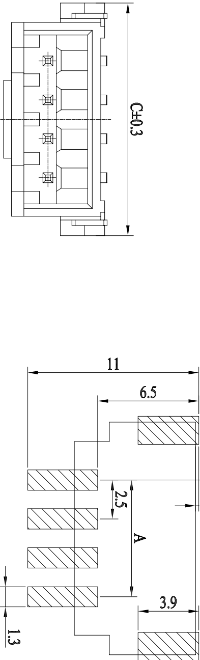
POB板安装尺寸
